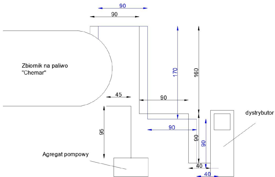
Rys 1. Schemat orurowania LPG (widok z boku)
